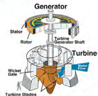
चित्र 11.26 : जेनेरेटरलाई तीव्र गतिमा घुमाउन प्रयोग हुने टर्बाइन
