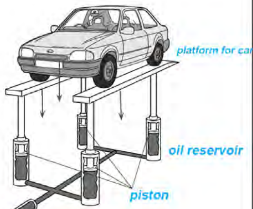
चित्र 8.15 हाइड्रोलिक कार लिफ्ट
