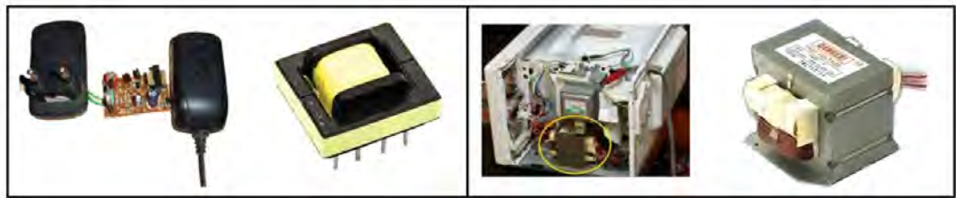
चित्र 11.30: चार्जरमा ट्रान्सफर्मरको प्रयोग
