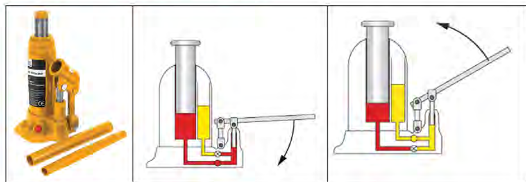
चित्र 8.17 हाइड्रोलिक ज्याक
