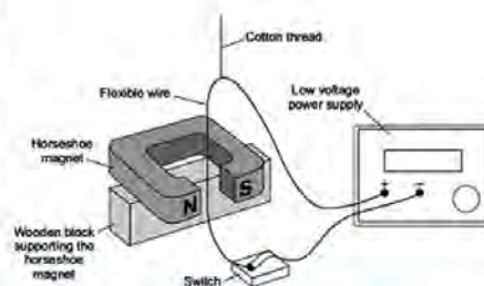
चित्र 11.23: मोटर असर प्रवर्तन
