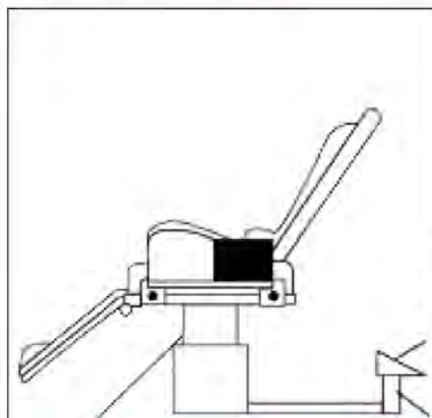
चित्र 8.14 पास्कलको नियमका आधारमा निर्माण भएको हाइड्रोलिक लिफ्ट
